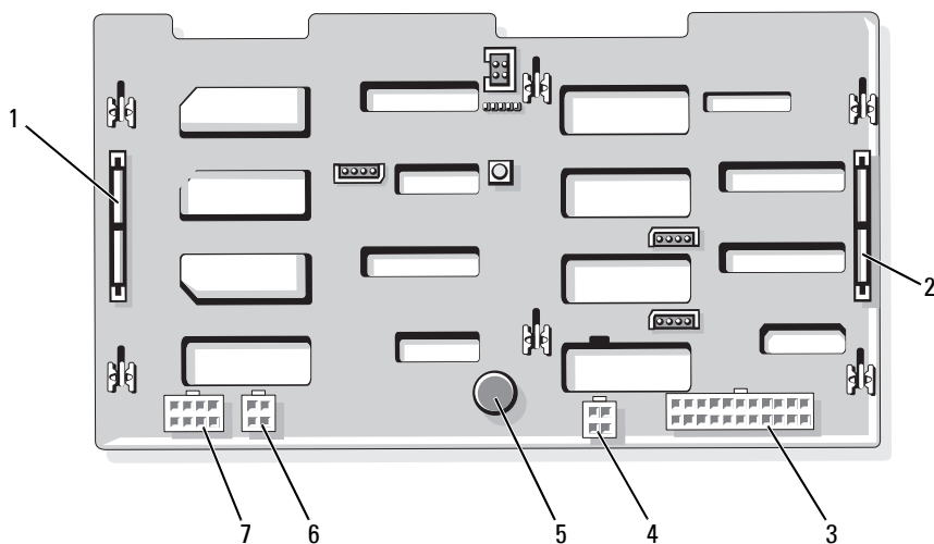
图 6-3. 1x8 SAS 背板连接器
