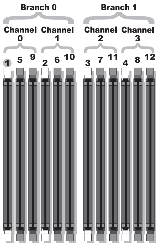
图 3-21. DIMM 插槽
