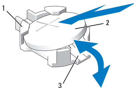
图 3-19. 更换系统电池
